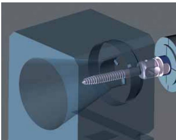
Simulation d'une opération de tourbillonnage pour la réalisation d'une vis à os.
