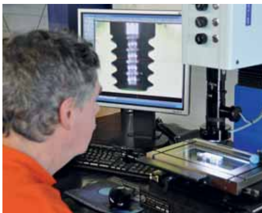
L'innovante tecnica permette di effettuare una misurazione ottica dei particolari ed i valori così ottenuti vengono analizzati dal sistema di controllo qualità con il soft QuickControlPro®.
