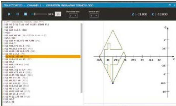
刀具轨迹模拟示例：网站图片
